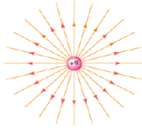
الف) خطوط میدان الکتریکی در جهت دور شدن از ذره باردار +q است.
