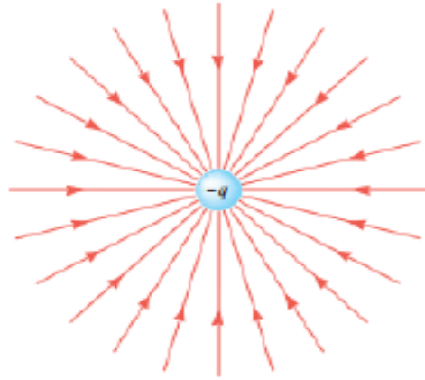
ب) خطوط میدان الکتریکی به سمت ذره باردار -q است.
